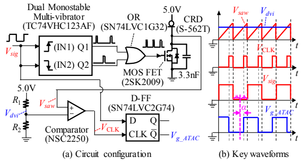
Fig. 10. Phase shift circuit.
