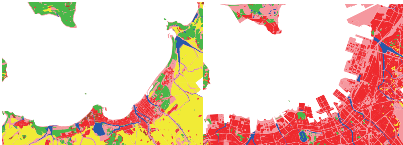
図 2-2 明治（左）と平成（右）の海岸線変化
