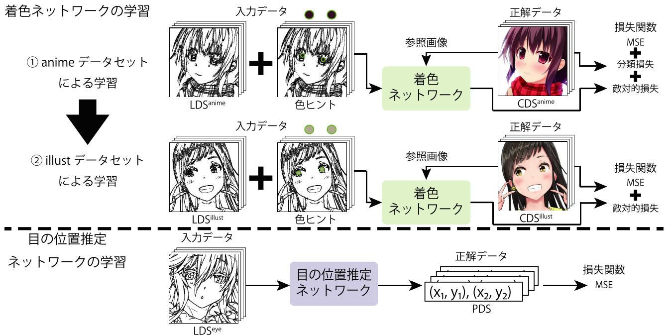
図 2 学習の概要図. 着色ネットワークは \mathcal{L}^{anime} と \mathcal{C}^{anime} での学習を行った後①, \mathcal{L}^{illust} と \mathcal{C}^{illust} の学習②を行う
