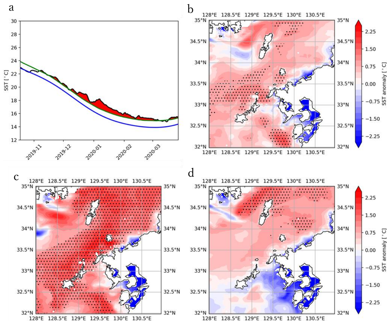
図 4.2 (a)は 2019 年 11 月から 2020 年 3 月にかけて海洋熱波が発生した期間の壱岐沖 (図 4.1a の赤丸) の海面水温の時間変化。赤で塗りつぶされた領域が海洋熱波の期間である。黒線は日別海面水温、青線は気候値、緑線は閾値を示す。(b)海洋熱波の発生初期(2019/12/04)、(c)水温偏差が最大に達した時期(2020/01/07)、(d)海洋熱波の終息時期(2020/03/16)における海面水温の水温偏差。黒のドットは海洋熱波が発生している箇所を示す。
