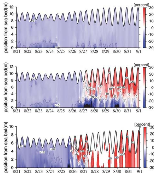
図 8 Case I に対する DO 増加率の計算結果 (上: Case III(A), B3.中: Case III(D), B3, \beta=6.4 .下: Case III(D), Sta.A, \beta=6.4 ) 12)
