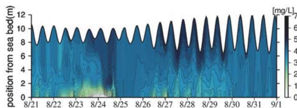
図 7 DO の計算結果(B6 地点, Case I) 12)
