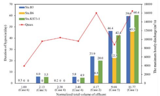
図 14 正規化した筑後川の総流出量に対する底層貧酸素の 持続時間との関係
