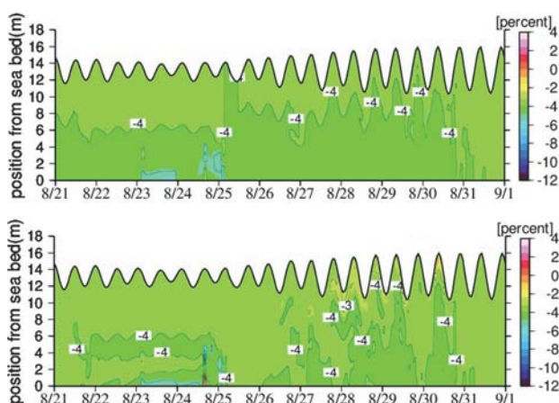
図 4 ケース①に対する DO 増加率の計算結果 (B6 地点. 上図: ケース②(A), 下図: ケース②(B)) 11)
