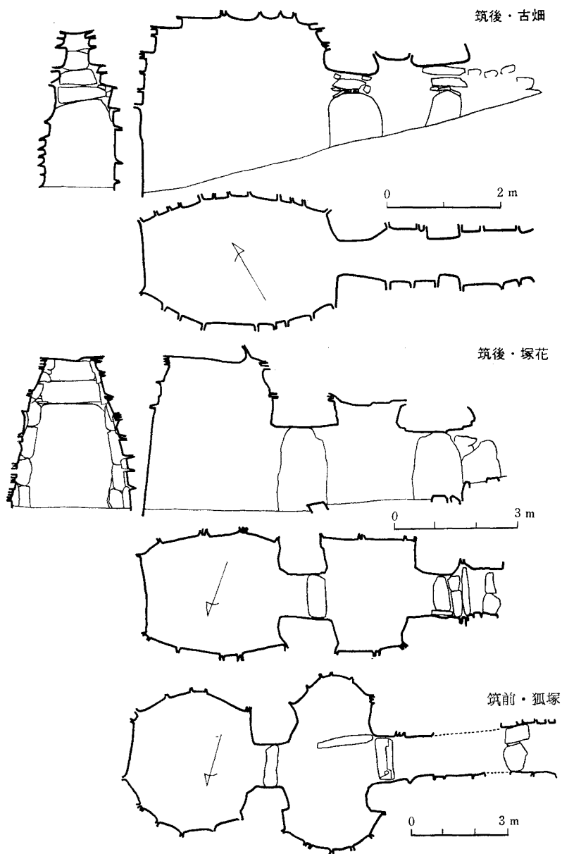
第 15 図 法恩寺山第三号古墳石室と類似構造を示す石室対照図
