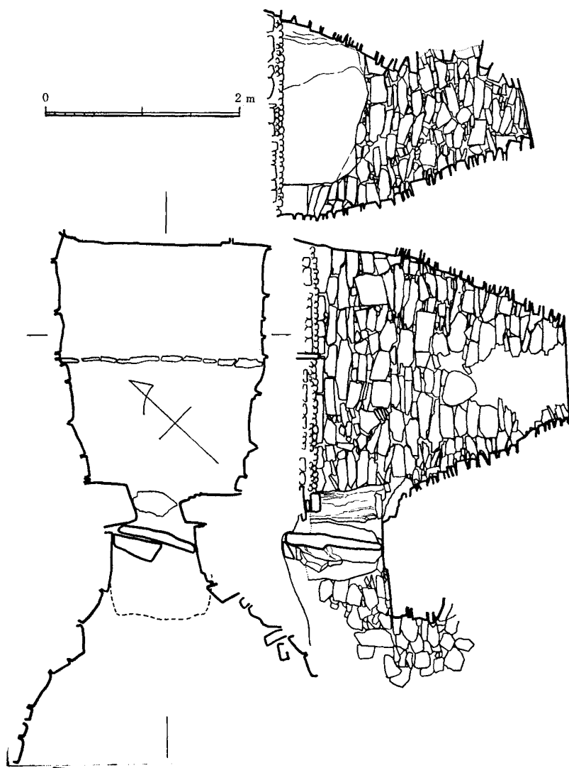
第11図 法恩寺山第四号古墳石室実測図
