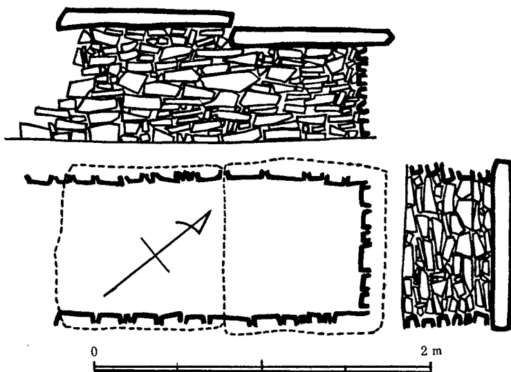
第 6 図 姫塚古墳石室実測図 (賀川光夫氏による)
