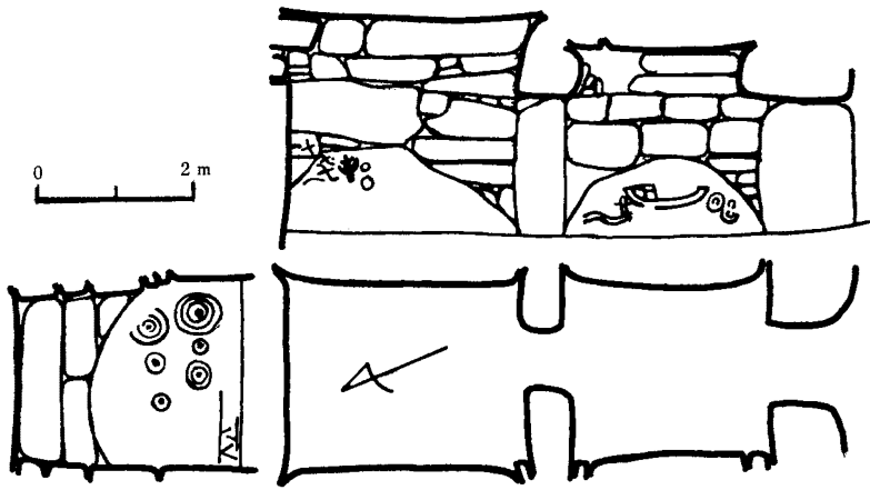
第13図 穴観音古墳石室実測図
