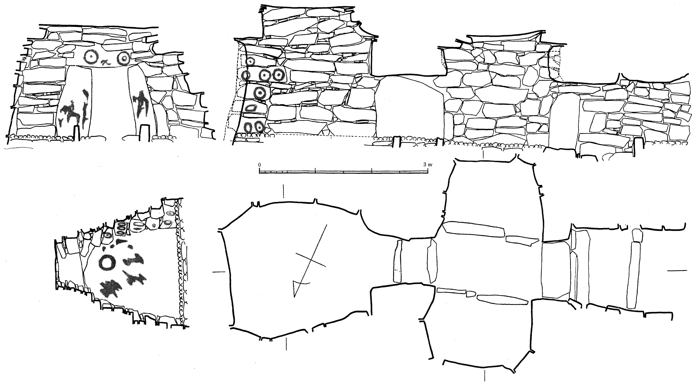
第10図 法恩寺山第三号古墳石室実測図（「法恩寺古墳」により一部修正）
