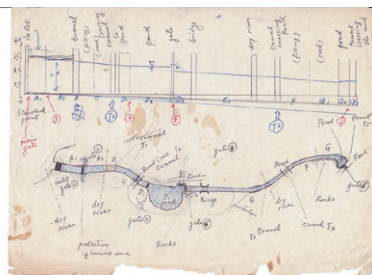
中村哲医師直筆 用水路概略図（2003）
