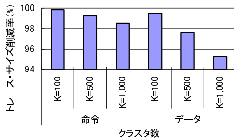
図 10 クラスタ数とトレース・サイズ削減率の関係 Fig. 10 Impact of K on trace size
