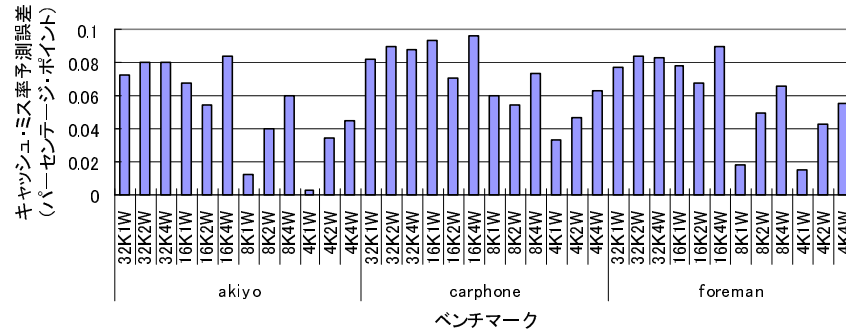
図 8 データキャッシュにおける MPEG2 のキャッシュ・ミス率予測誤差
