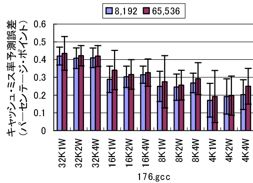
図 14 データキャッシュにおけるアドレス・インターバルと精度の関係
