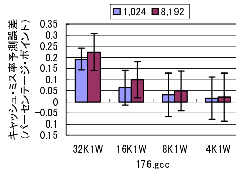
図 13 命令キャッシュにおけるアドレス・インターバルと精度の関係 Fig. 13 Impact of address-interval size on accuracy (I-cache)
