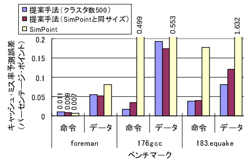
図 16 SimPoint とのキャッシュ・ミス率予測誤差の比較
