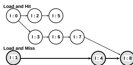
図3 クリティカルパスの変化 Fig.3 Exchange of the Critical Path
