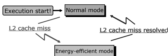
図 6 モードの切り替わり Fig. 6 Mode Transition
