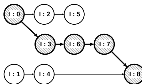
図 1 クリティカルパス Fig. 1 Critical Path
