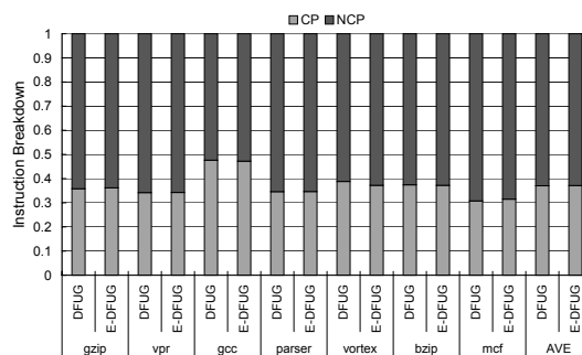
図10 省電力モード中の命令の内訳
