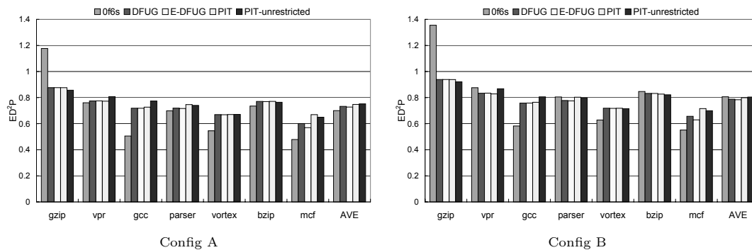
図 11 エネルギーへの影響 Fig.11 Energy-Efficiency Results
