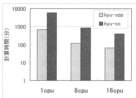
図 4 : 日本海モデルの1年間の計算時間の比較 (対数目盛である事に注意)。
