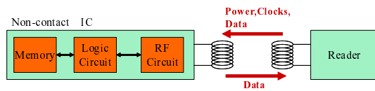
Fig.1 An RFID tag
