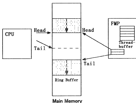
図5 実行可能スレッド待ち行列 Fig. 5 Thread Queue.
