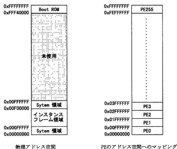
図7 メモリマップ Fig. 7 Memory map.
