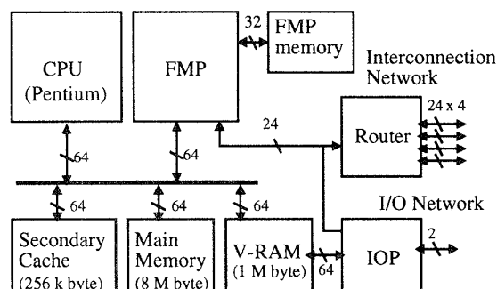
図 2 プロセッサエレメント
