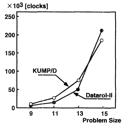
図10 fibonacci (n) の実行時間
