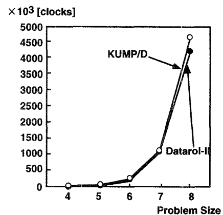
図11 Queen (n) の実行時間
