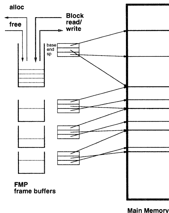
図6 インスタンスフレーム管理 Fig. 6 Instance frame stuck.
