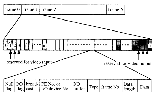
図 9 Video Frame の分割
