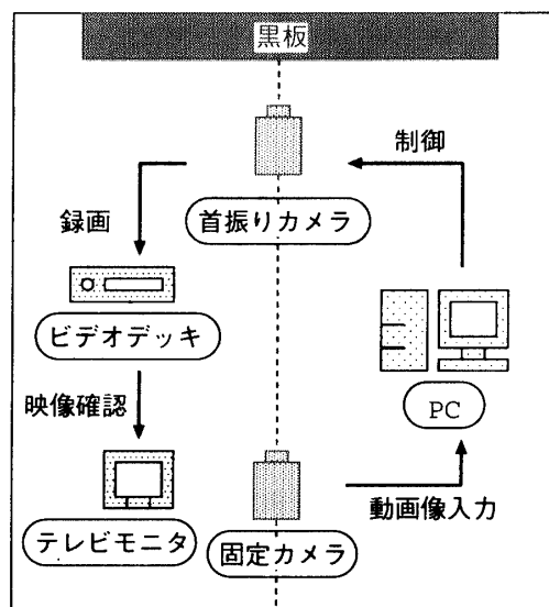
図 6: 実験環境
