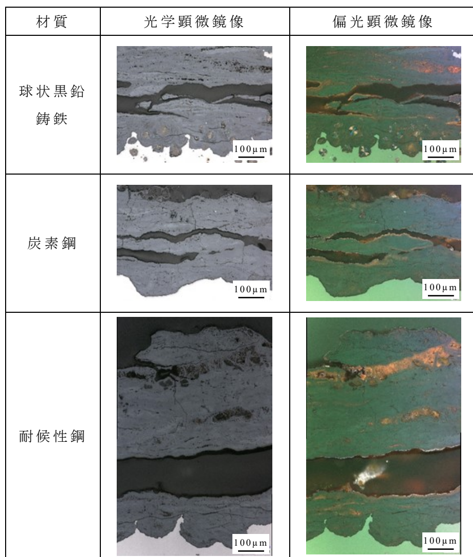
図 4-5 さび層断面の光学顕微鏡像および偏光顕微鏡像（百道／4年暴露後）
