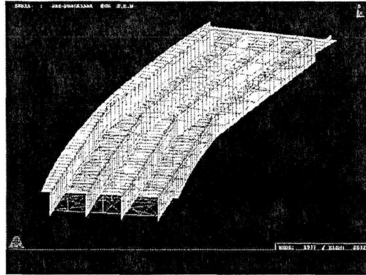
図 1: 橋梁の間の有限要素法メッシュ図 (行列: BEAM).
