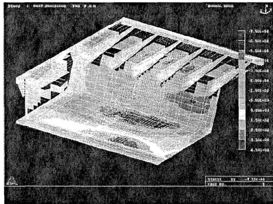
図 5: 応力 ( x - y 方向成分) 分布 (行列: CABLE)。
