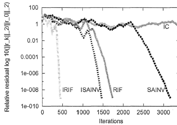
図 3: 行列: BEAM に対する IC 分解, RIF および IRIF 前処理つき CG 法の収束履歴.
