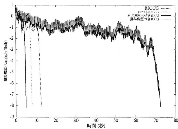
図 4: (同行列) 重み調整 IC, RIC, pf-RIC および対角緩和 RIC 前処理つき CG 法の収束履歴.
