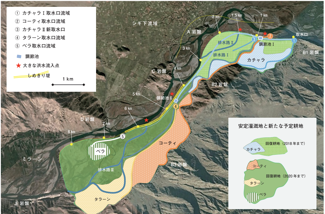
主な既存灌漑用水路と各流域
