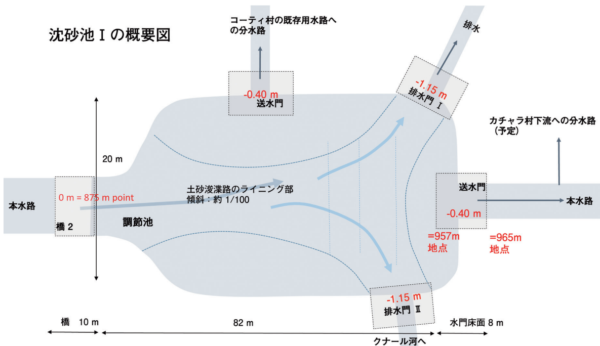
沈砂池概要図。マルワリードⅡ用水路約900m地点にあり、本水路への送水門、コーティ村への送水門と2つの排水門を備える。
