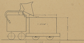
ロッガーショベルと木製炭車の積込関係図
