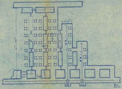
(柱房式) 採炭規格圖 (掘却式)
