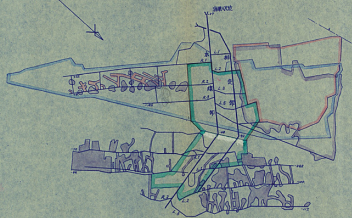
海八坑 坑內圖 S=3000 分/1
