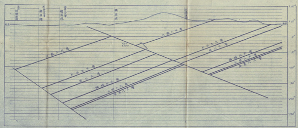
C-D 截断面圖
