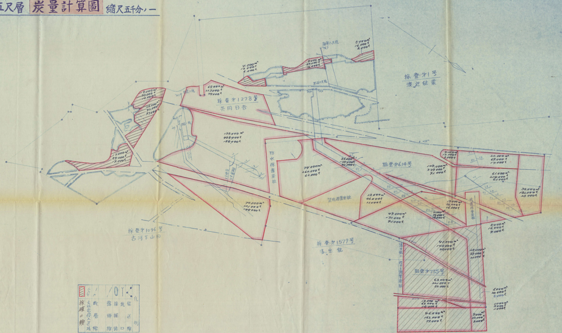
蝙蝠五尺層 炭量計算圖 縮尺五千分、一
