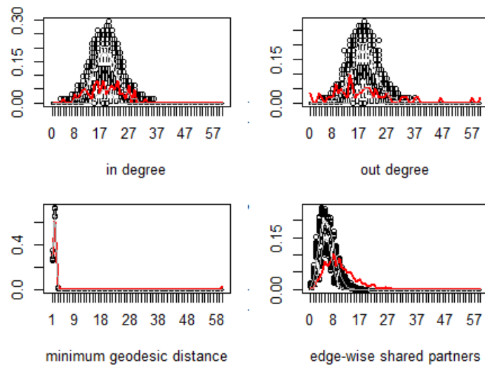
Figure2 モデル1のBGOF
