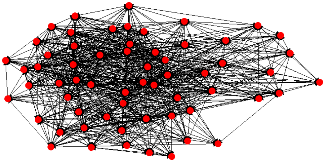
Figure1. 観測されたネットワーク
