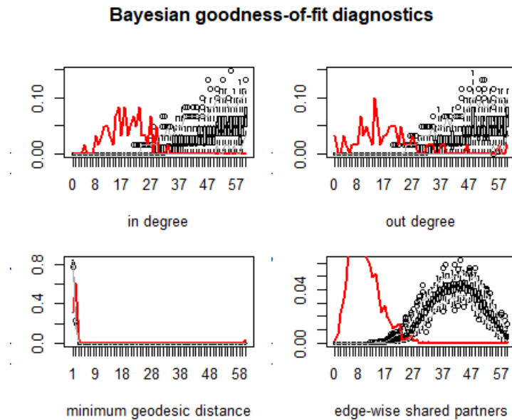
Figure4 モデル3のBGOF
