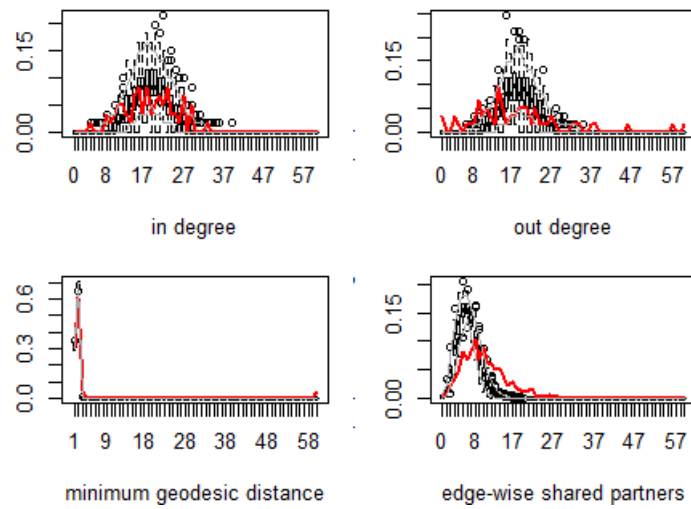
Figure3 モデル2のBGOF
