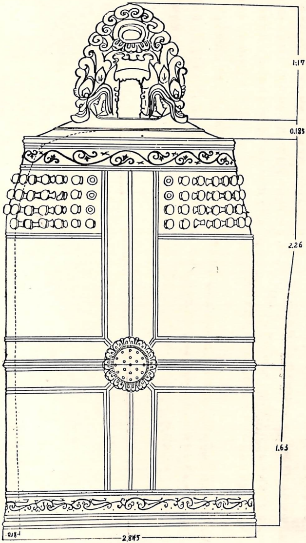
圖版十一 觀世音寺鐘 實測圖（昭和廿六・九・廿四作製）
