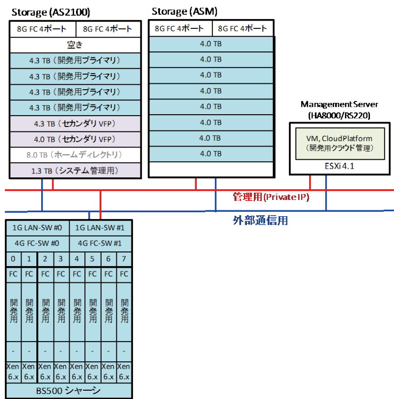
参考資料 1 キャンパスクラウドシステム構成図
