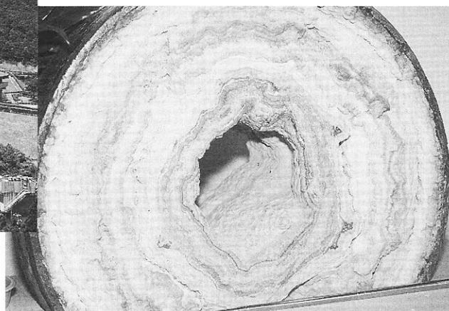
↑ 永く使用した蒸気井のパイプ
