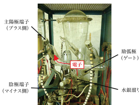
水銀整流器近影(2015年5月26日筆者撮影)
