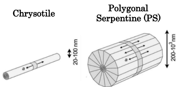
図 1 Chrysotile 及び PS の結晶構造の模式図 (Cressey et al. 2010 を改編)
