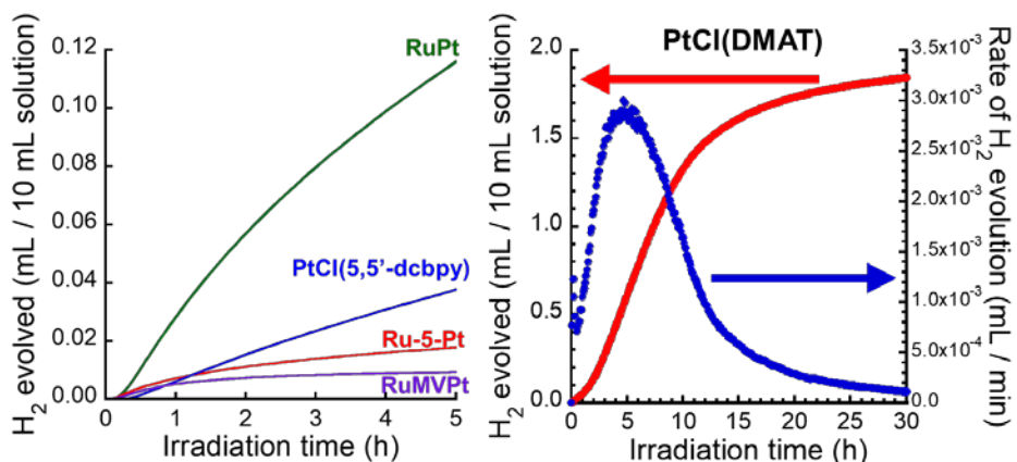
図 1. RuPt 系及び Pt 系単分子光水素生成デバイスの光水素生成挙動 (錯体濃度:0.1 mM、pH5.0、20°C、30 mM EDTA 共存下)
