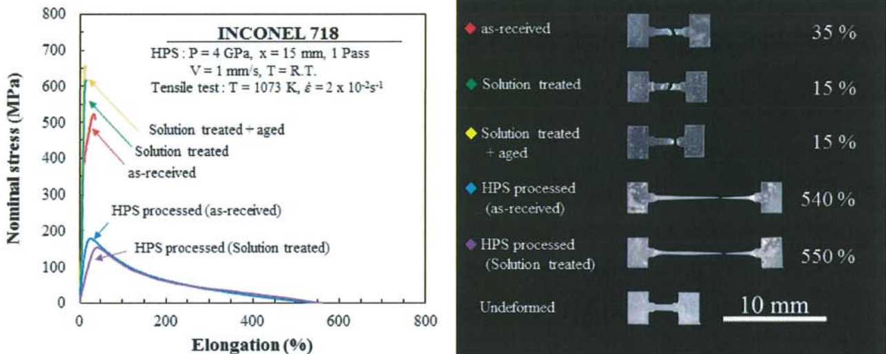
Fig. 1 受領材と受領材の熱処理材(溶体化、溶体化+時効)、HPS 加工材(受領材および溶体化材) を試験温度 1073 K、初期ひずみ速度 2 \times 10^{-2} s^{-1} で引張破断させた際の応力-ひずみ曲線(左)と引張試験前後の試験片外観(右)
