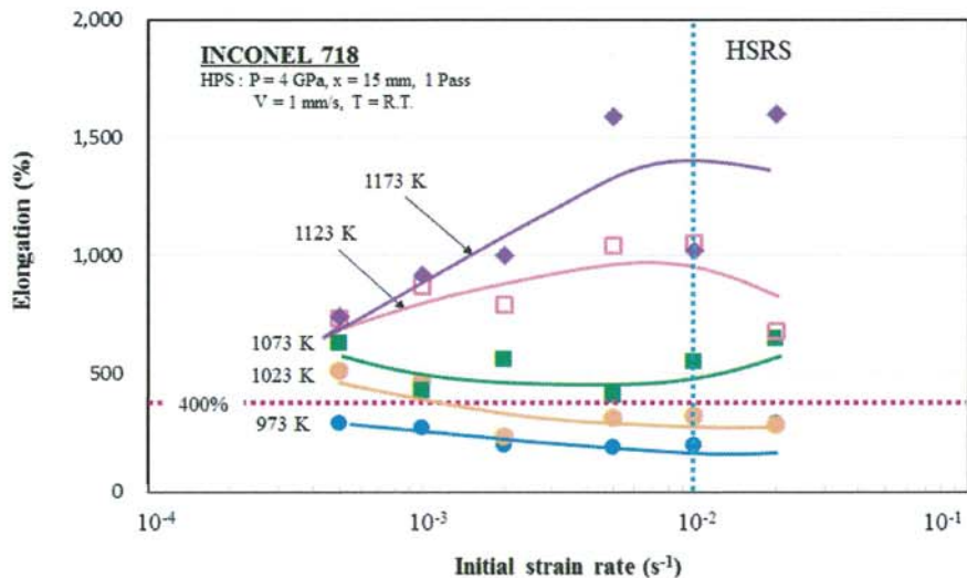
Fig. 2 試験温度 973~1173 K におけるひずみ速度と伸びの関係
