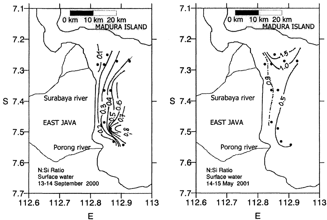
Fig. 13 N:Si ratio
