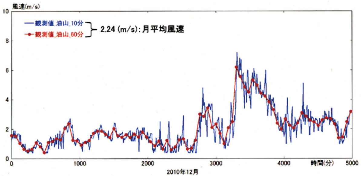
図5 時間解像度(10分および60分)の比較, 油山地点, 地上高10m
