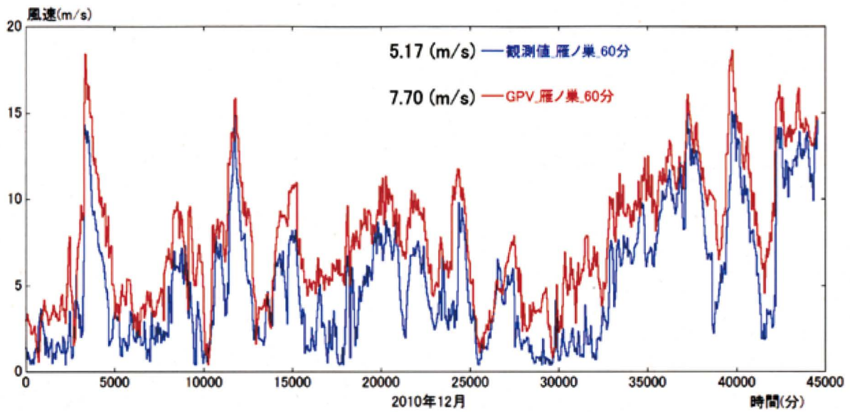
図6 野外觀測データと気象GPVデータ(MSM-S)の比較, 雁ノ巣地点, 地上高10m
