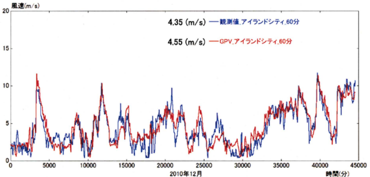
図7 野外觀測データと気象GPVデータ(MSM-S)の比較, アイランドシティ地点, 地上高10m
