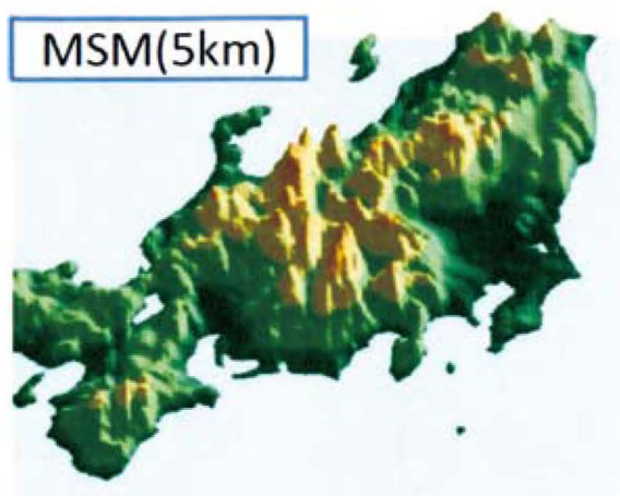
図2 MSMの地形解像度
