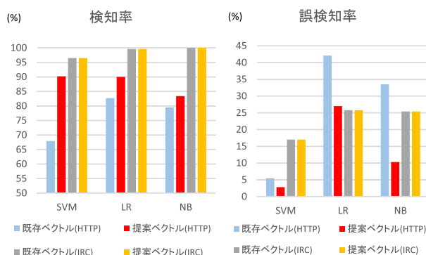
図7 提案ベクトル、既存ベクトルとの比較に関する実験結果
