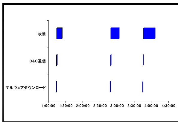
図 1 ボットネット活動の時系列調査
