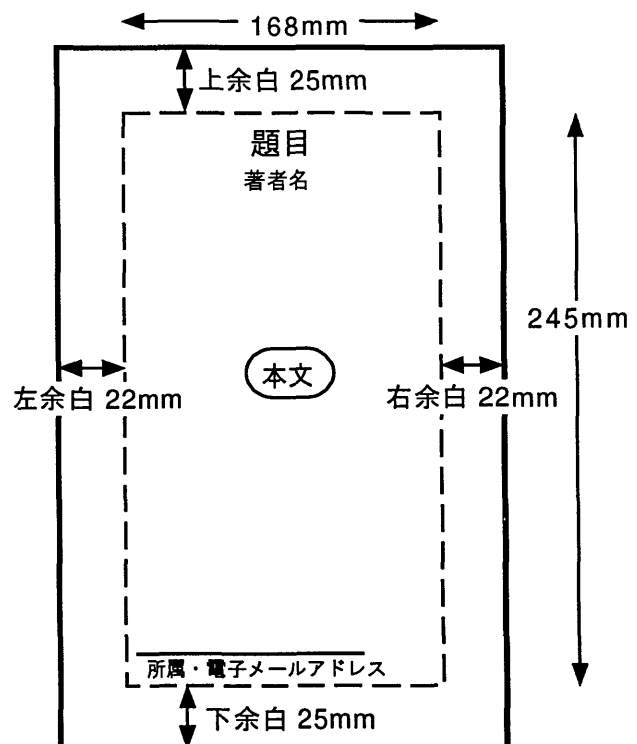
図 1: 書式設定
