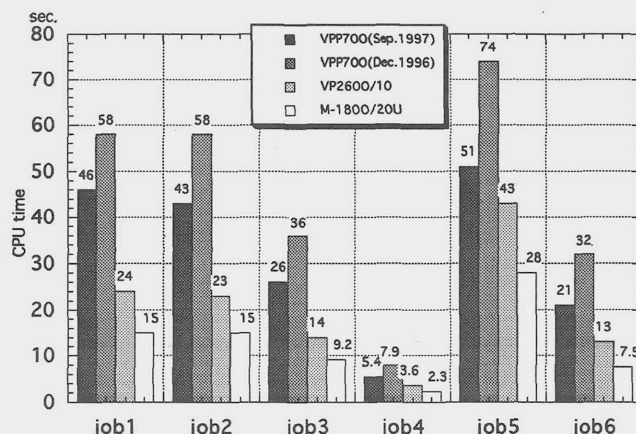
図1: 翻訳性能の比較 (表2のグラフ)
