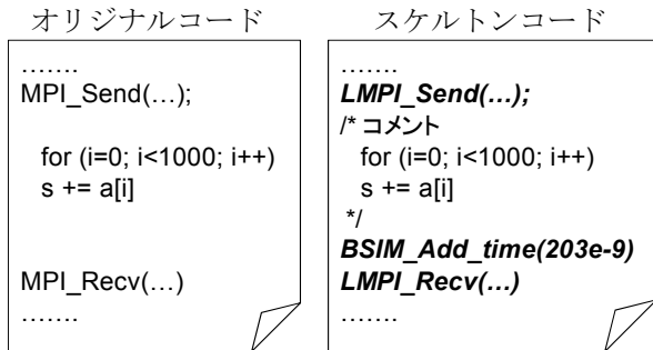
図 2：スケルトンコード
