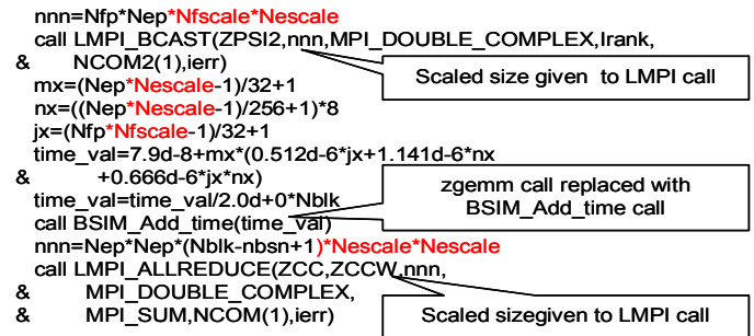
図 3：スケルトンコードの実例（PHASE の一部）
