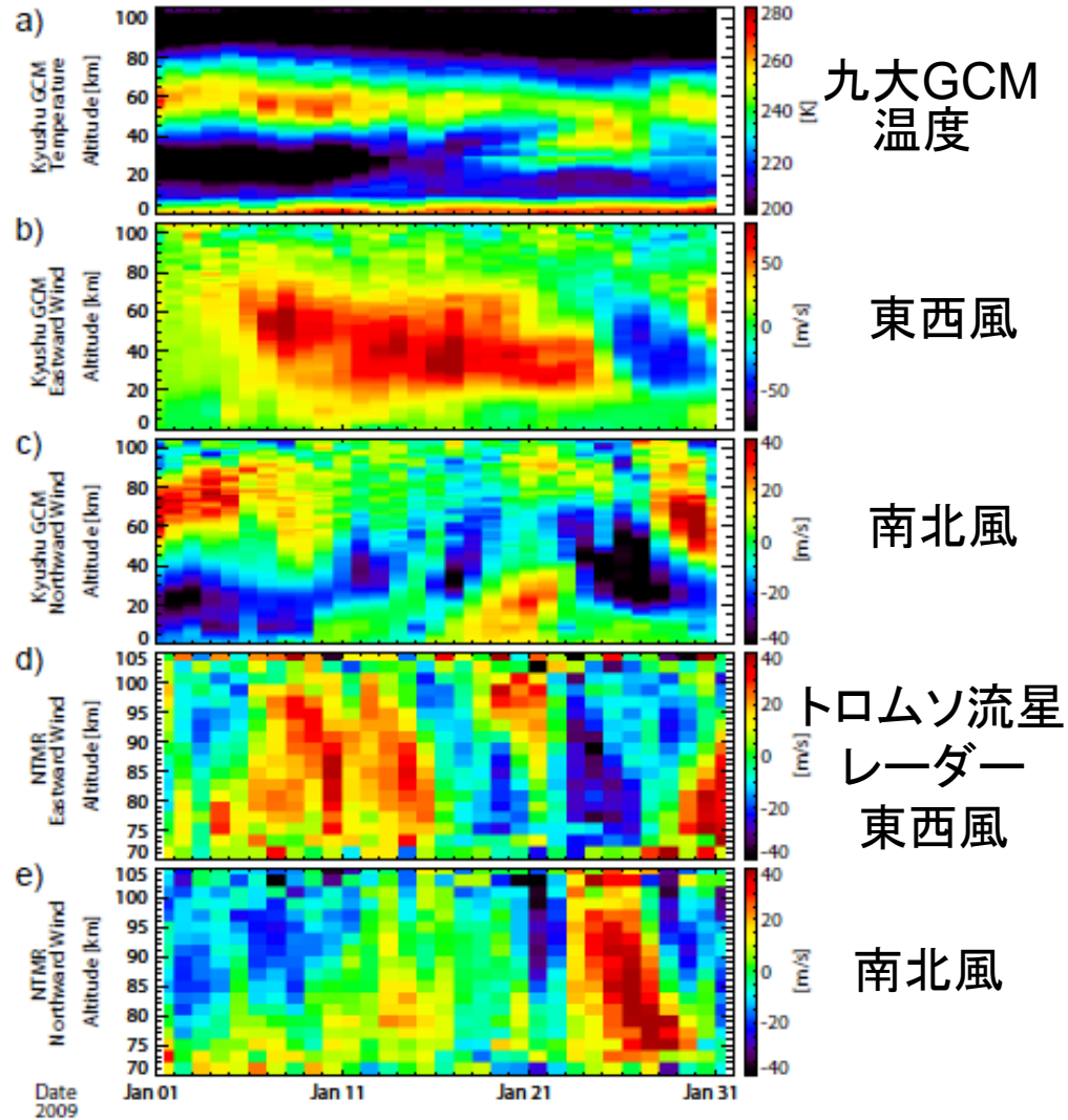
2009年1月の成層圏突然昇温時の九大GCMとトロムソ流星レーダーの比較
